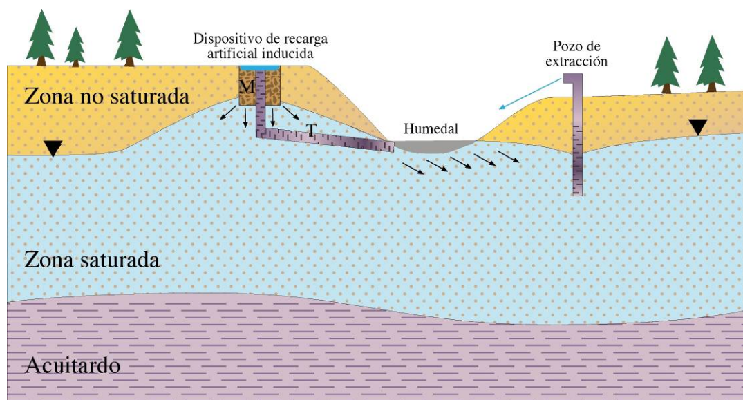
Figura 8. Diseño genérico de un dispositivo de recarga artificial inducida para aumentar la salinidad de las aguas de recarga artificial hasta alcanzar unas características similares a las aguas indígenas regulando la superficie de contacto y el tiempo de interacción con el material salino natural del terreno, precipitado por el ascenso de flujos subterráneos profundos. Fdez. Escalante, 2005.
