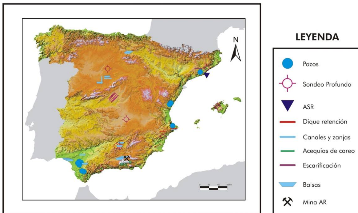
Figura 2. Principales estructuras y dispositivos de MAR operativos en España y tipologías.
