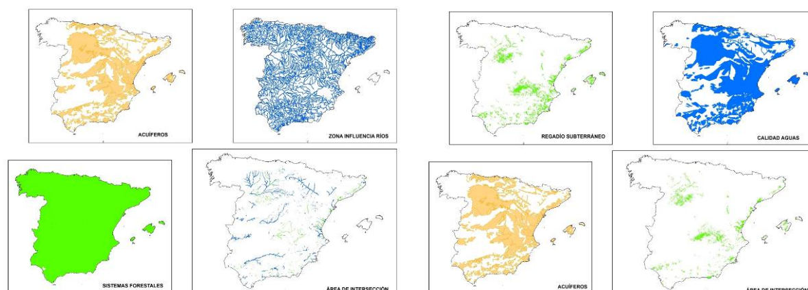
Figuras 9 a) a g). Imágenes de los primeros cruces de coberturas temáticas realizados con objeto de determinar las zonas (provisionales) susceptibles de regeneración hídrica en España.
