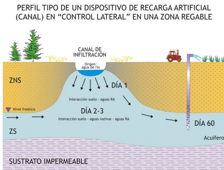
Figura 1. Esquema operativo de un dispositivo de recarga artificial de acuíferos (canal) en una zona regable.
