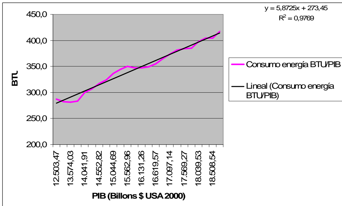
Figura 3.- Relación PIB mundial consumo de energía
