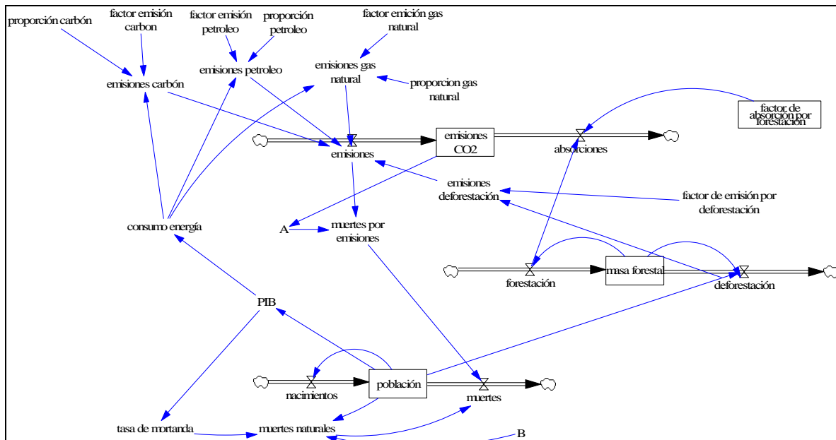
Figura 1.- Diagrama causal del modelo de emisiones y absorciones
